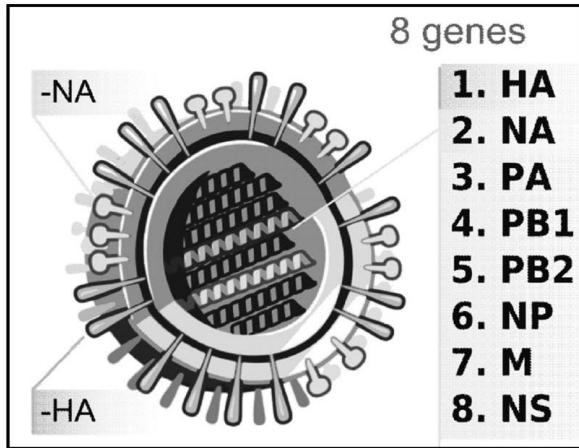
ภาพที่ 2 ส่วนประกอบของไวรัสใช้หัดใหญ่ ตัวอักษรย่อที่เห็นทางฝั่งขวา คือชื่อของยีนทั้งแปดชุด ซึ่งยีน HA เป็นตัวที่สร้างอีแอมกกลูตินิน และยีน NA เป็นตัวที่สร้างนิวรามินิเดสซึ่งทั้งคู่จะปรากฏบนผิวของไวรัส (แสดงเป็นตัวย่อทาง ฝั่งซ้าย) ที่มา: Wikimedia Commons (public domain)
